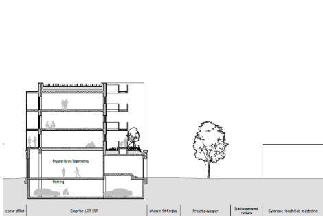
Coupe transversale rue Eymard Duverney
